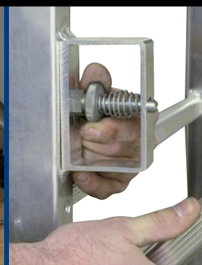
Mehanizam za zaključavanje pomoću opruge
